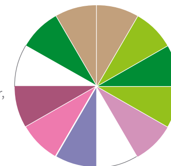
Farbspektrum
